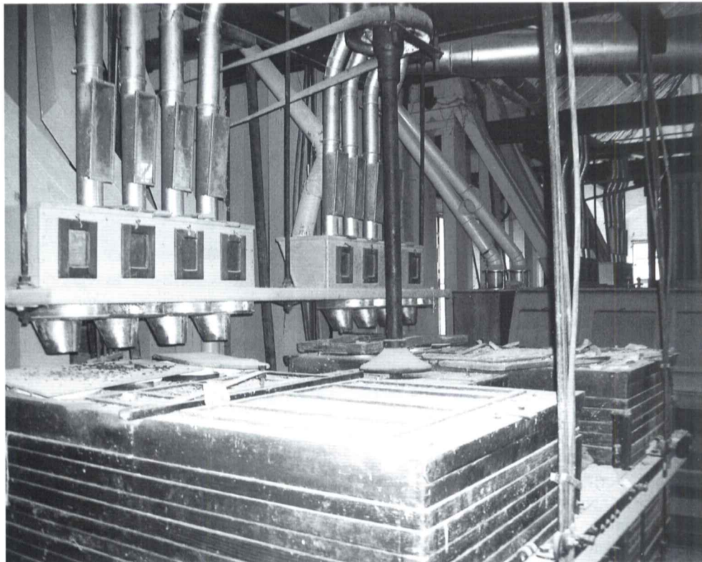
"Planschichter". Es un cernedor de libre oscilación que trabaja en sentido plano y circular con el mando de accionamiento central
