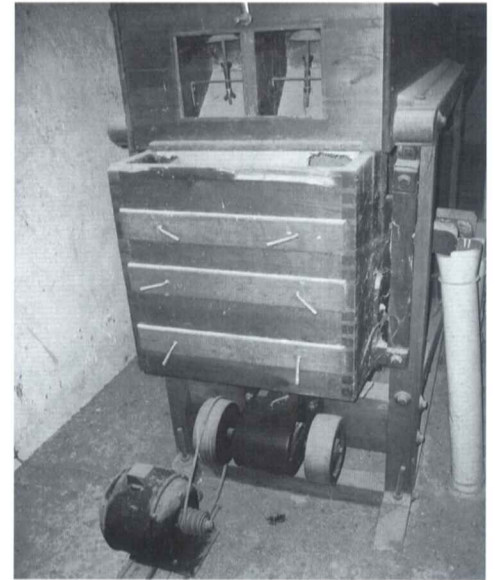
"Monitor". Generalmente es una de las primeras máquinas de la sección de limpia, consta de una caja que actúa como zaranda
