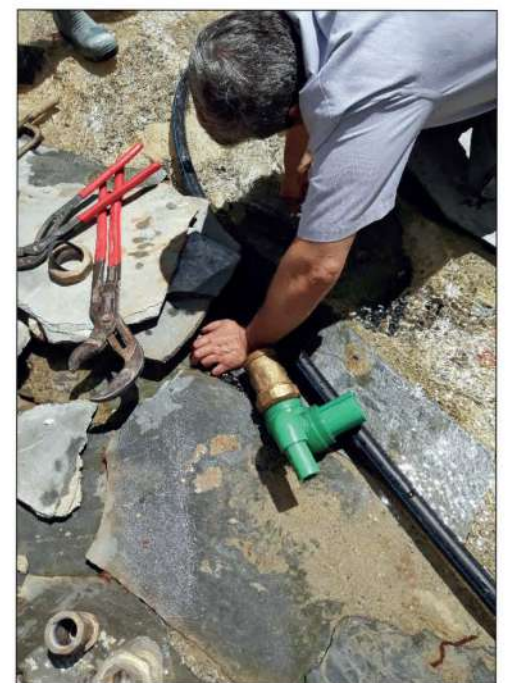
Trabajando en las filtraciones
